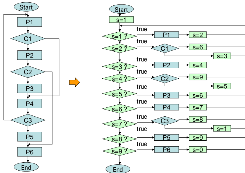
(紫合) 図2.8 構造化原理: 任意のプログラムは選択の繰返しにできる
