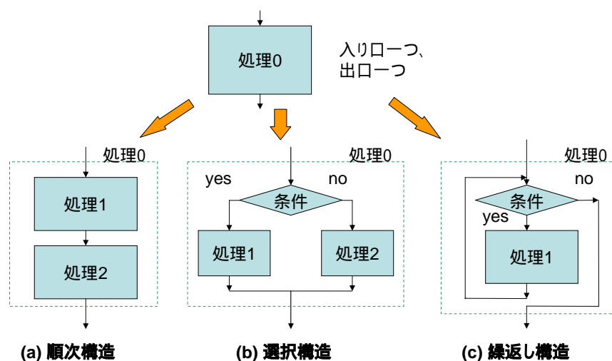
図1 処理と3基本制御構造による(1段階の)詳細化
