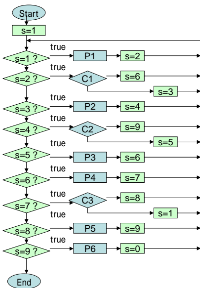
拡張構造化プログラミングによる書き換え例 (多分岐選択)
