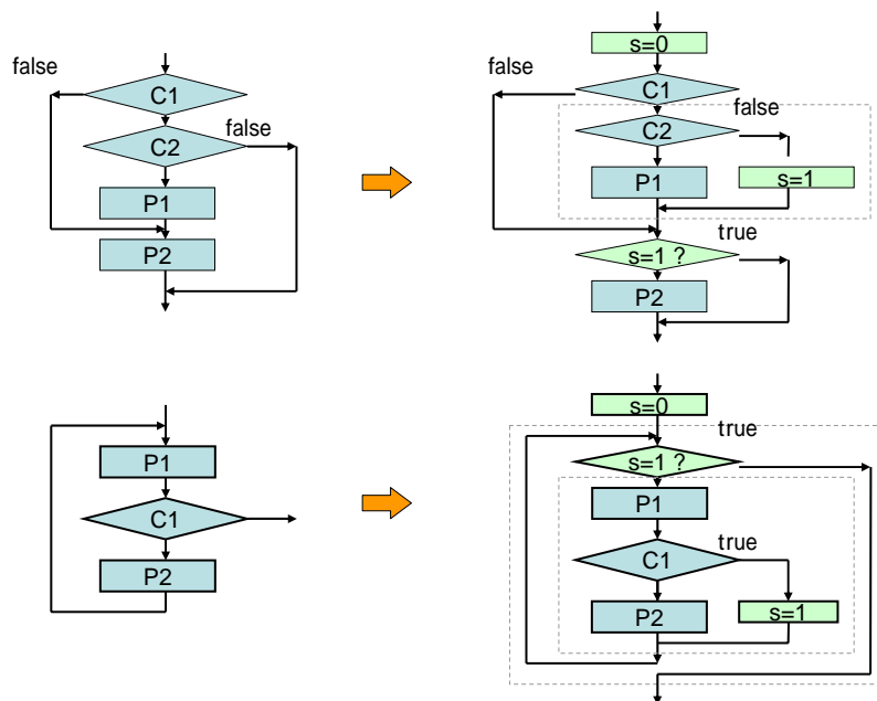
(紫台) 図2.7 構造化への変換 (制御変数による)
