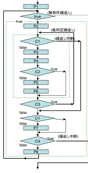
図2b 拡張構造化プログラミング を用いて書き換えた例
