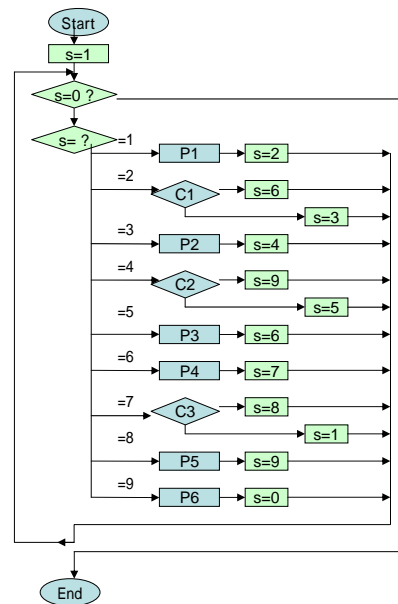
拡張構造化プログラミングによる書き換え例 (多分岐選択)
