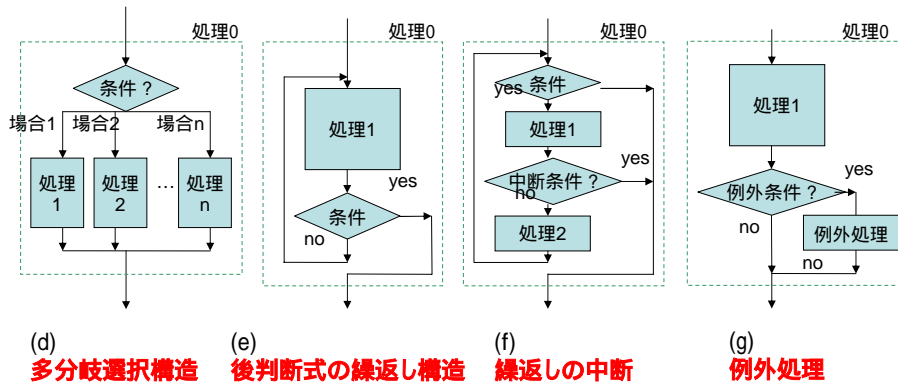
図2 追加の制御構造
