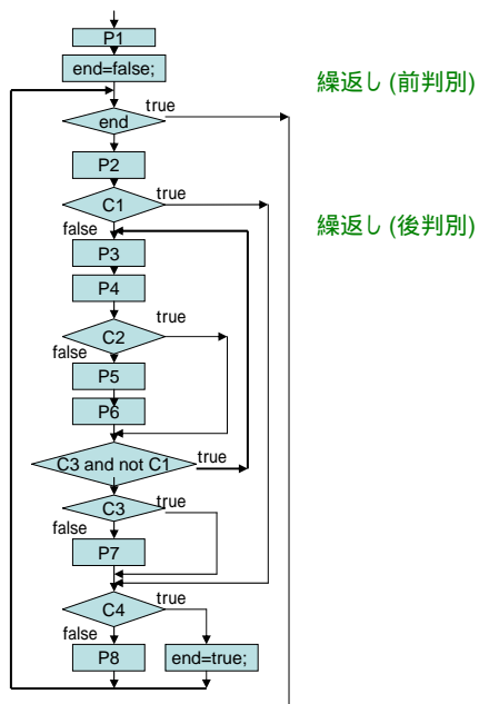
(紫合) 図2.5 等価な構造化プログラム (の例)
