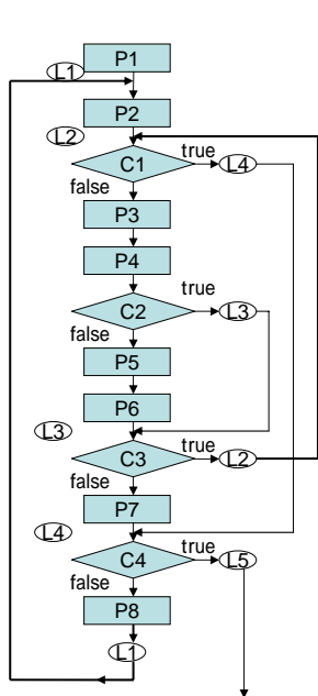
(紫合) 図2.4 Goto文を使った スパゲティプログラム (の例)
