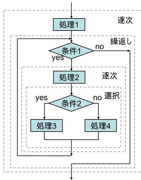
(紫合) 図2.3 基本制御構造の組合せ (の例)
