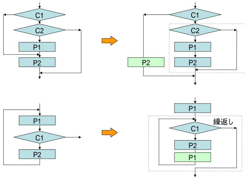
(紫台) 図2.6 構造化への変換 (処理のコピーによる)
