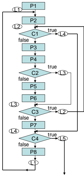
図2.4 Goto文を使った スパゲティプログラム (の例)
